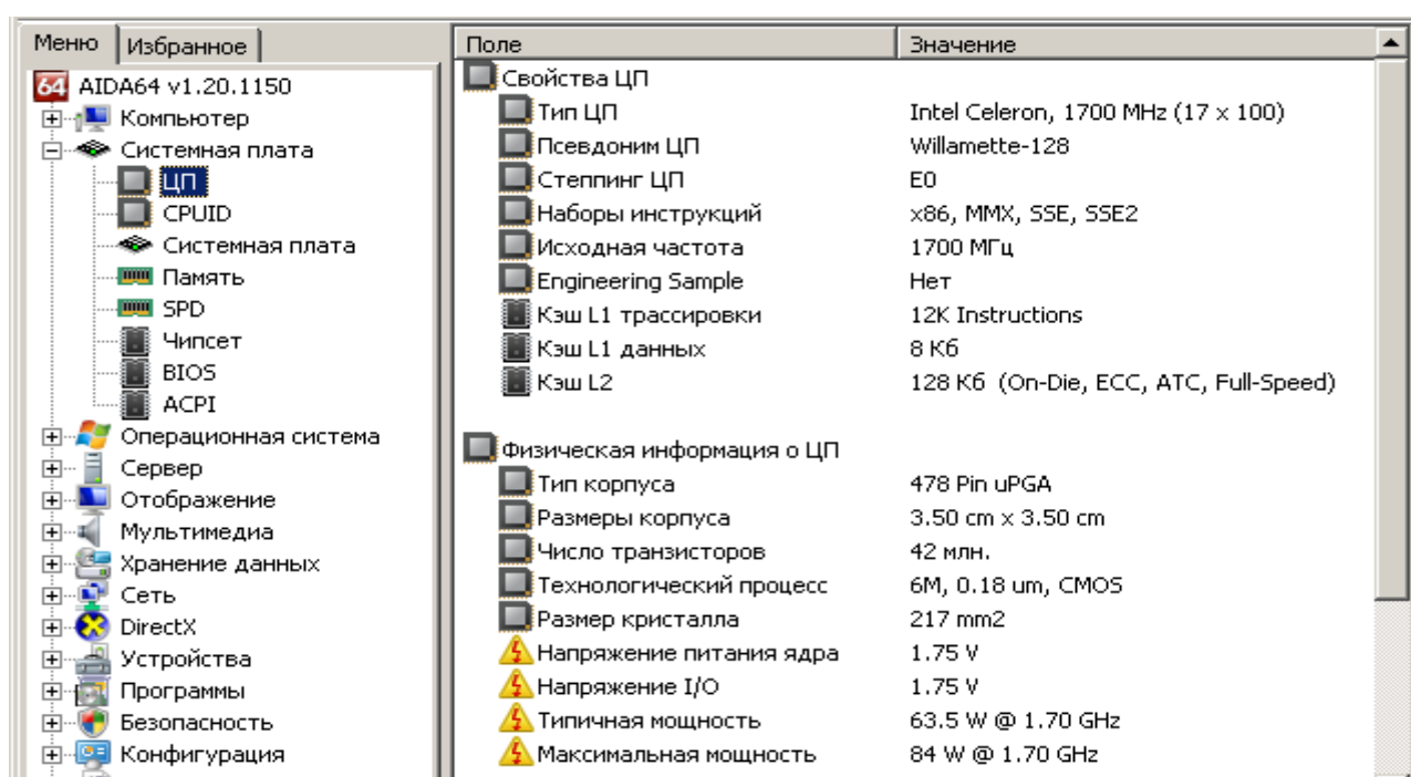
Рис. Ж.2. Відомості про центральний процесор
